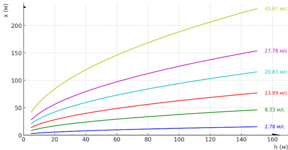
Рис. 2. Зависимость расстояния ( h ) между БПЛС и требуемой точкой приземления груза от скорости и высоты его падения ( x ) Fig. 2. Dependence of the distance ( h ) between the UAV and the required location of the load landing point on the fall velocity and altitude
