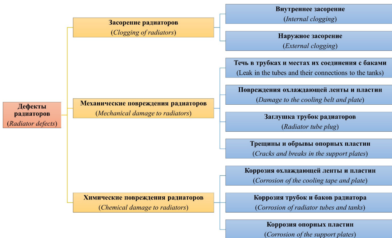
Рис. 4. Классификация дефектов радиаторов системы охлаждения ДВС
