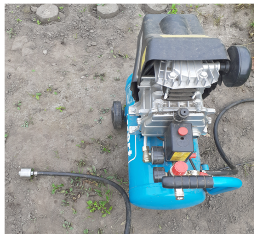
Рис. 2. Газоструйный излучатель, соединенный с компрессором Wert
