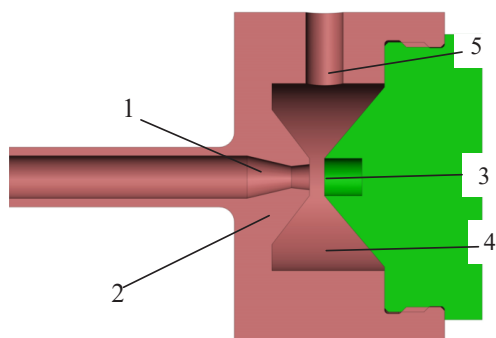
Рис. 1. Разработанный газоструйный излучатель:
