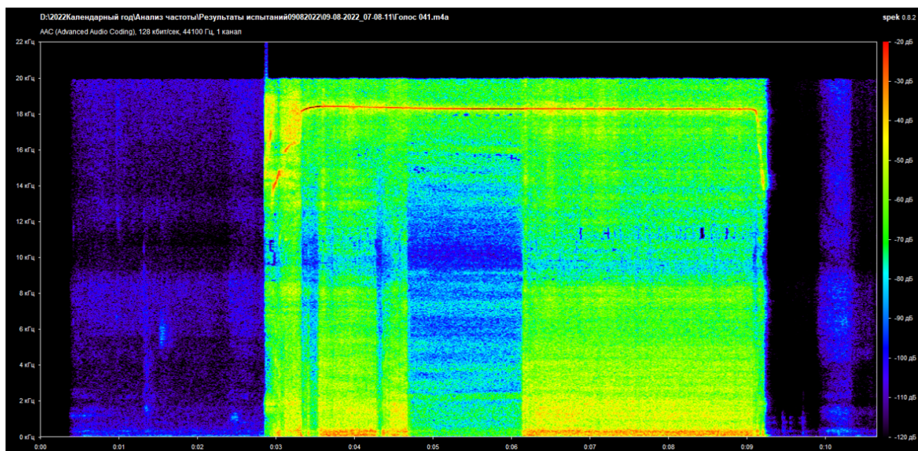
Рис. 3. Спектрограмма при расстоянии между соплом и резонатором газоструйного излучателя 3,75 мм и давлении сброса ресивера 4 МПа
