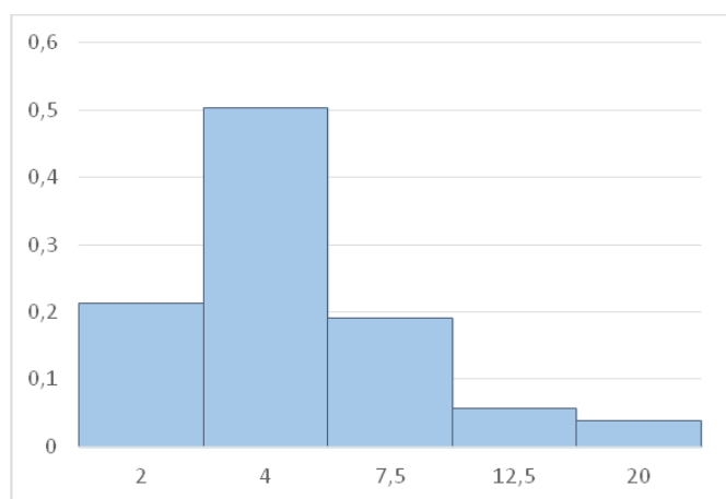
Рис. 2. Гистограмма распределения
